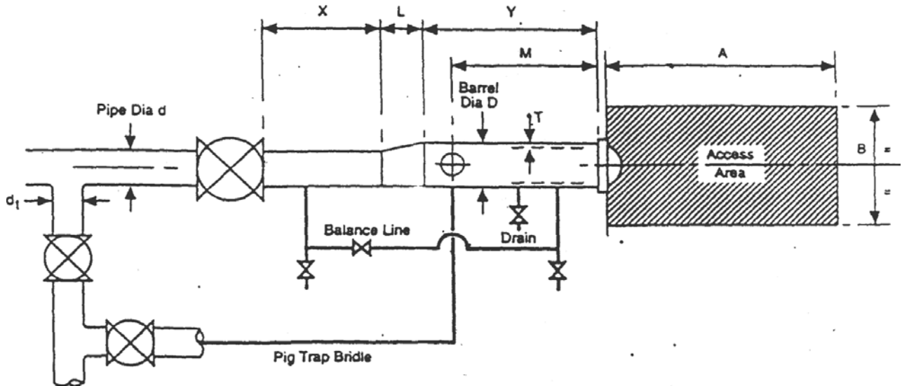
Типова схема на пускова/приемна камера
